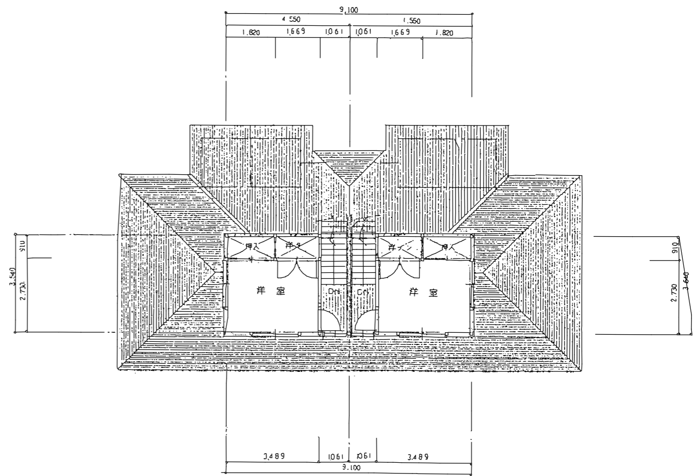
2楼平面图 S=1:100
