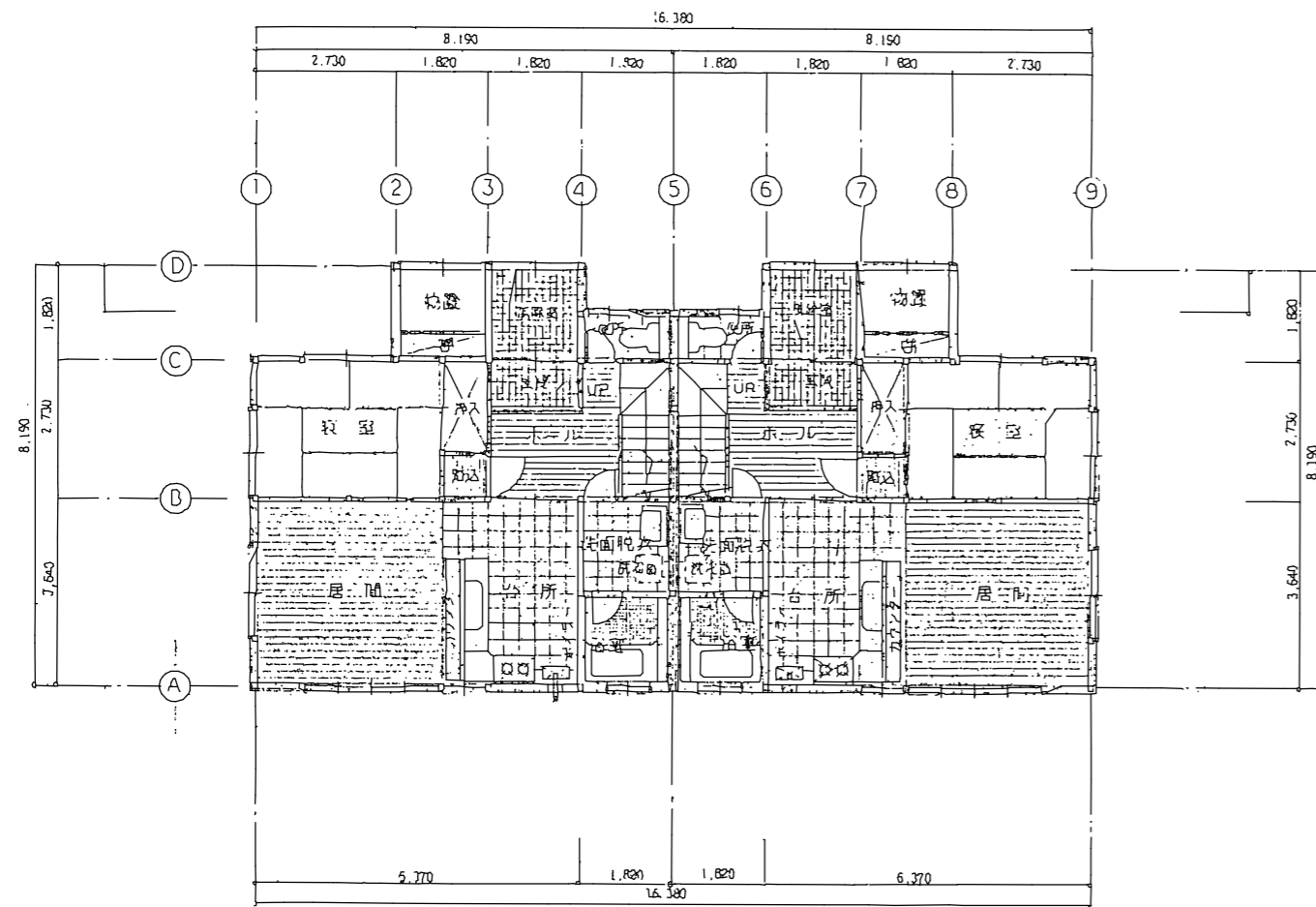
1楼平面图 S=1:100
