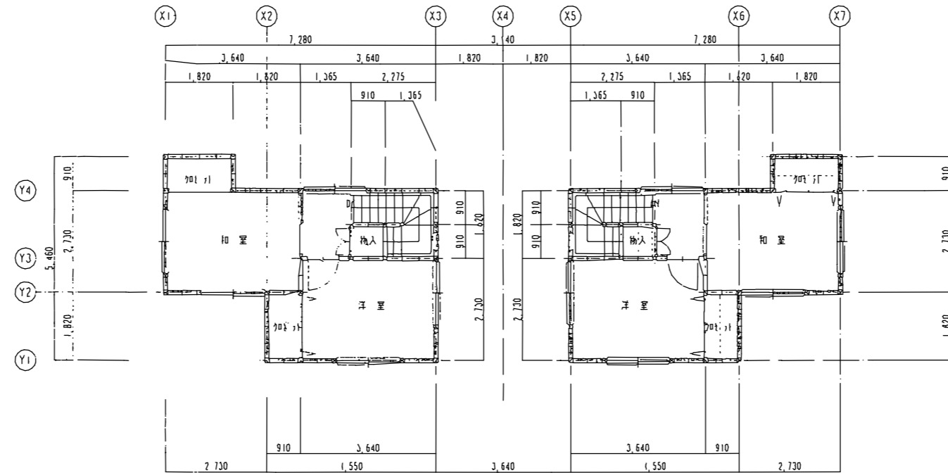
2階平面図 1/100
