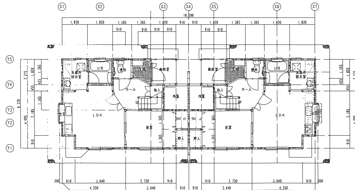
1階平面図 1/100
